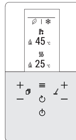
fig. 2 - interfaccia utente
